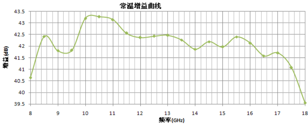
8~18GHz 宽带功放测试数据
